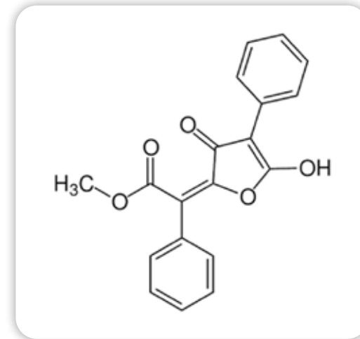
Strukturformel Vulpinsäure
